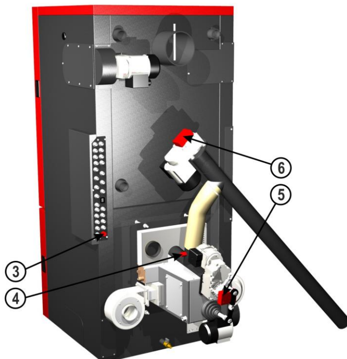
Obr. č. 2 Umístění prvků termostátů a snímačů otáček
