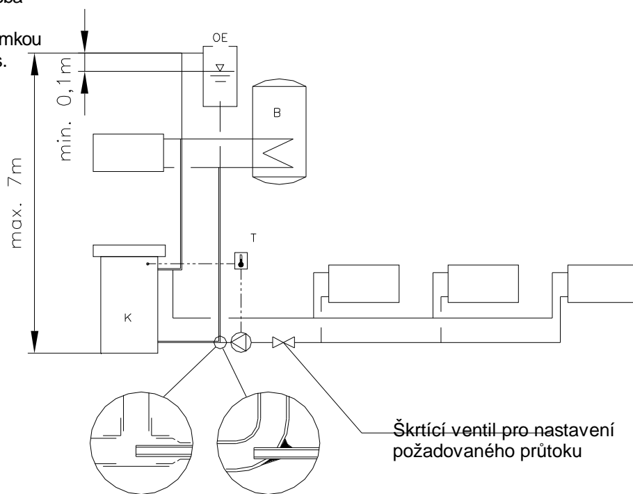
PŘÍKLADY ZAPOJENÍ
